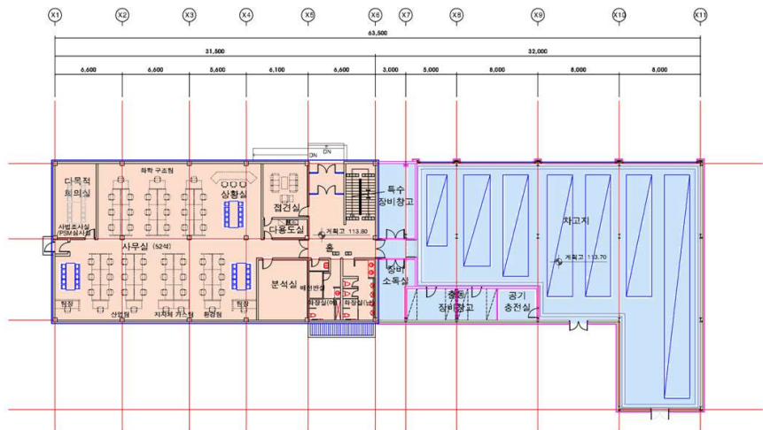
[지상1층 평면도]
