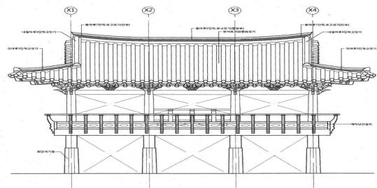
정면도(안)
