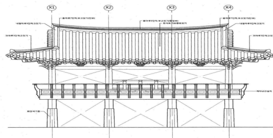
정면도(안)
