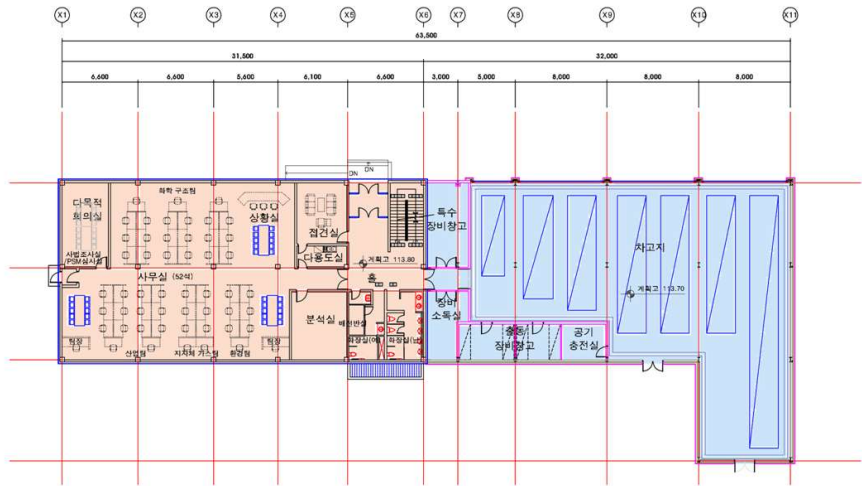
[지상1층 평면도]
