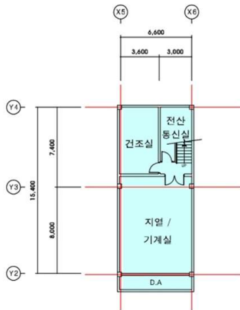
[지하1층 평면도]
